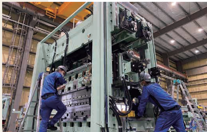
▲大型自動省力化ラインを代表とする専用機の組み立て作業の様子
